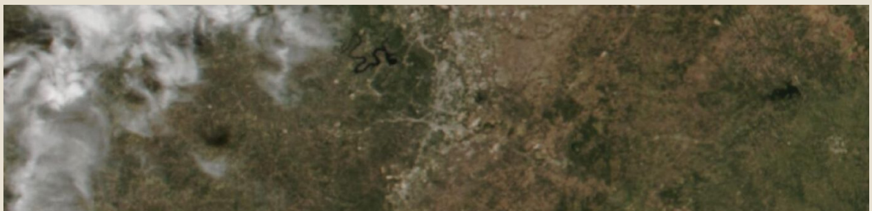
NASA Worldview · Austin, Vereinigte Staaten von Amerika · 22.10.2026
